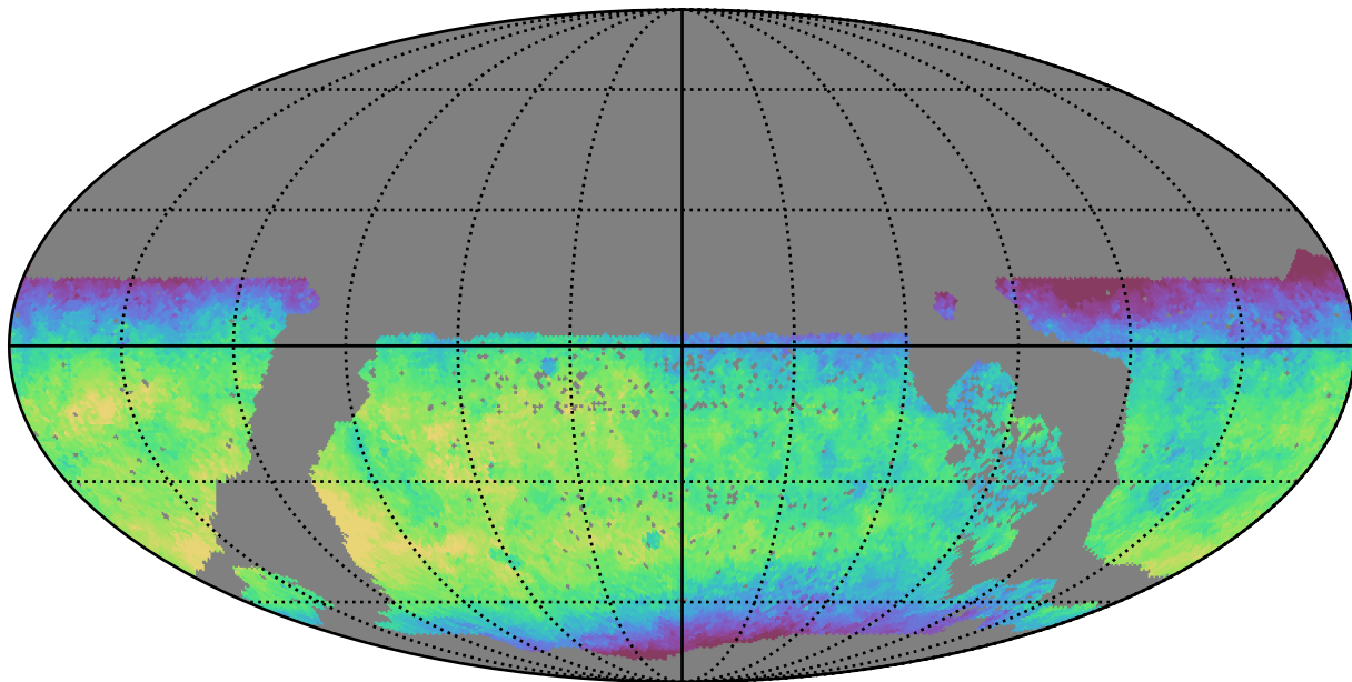
roman_v3.3_10yrs WFD y band: Median fiveSigmaDepth
