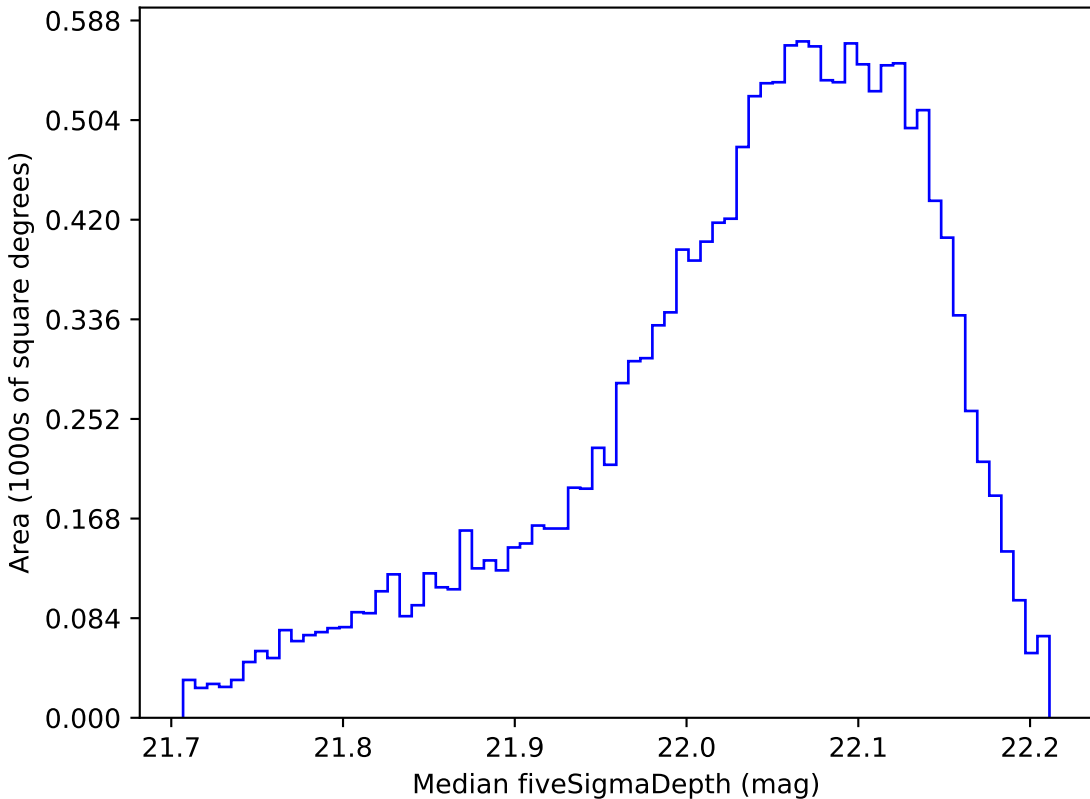
roman_v3.3_10yrs WFD y band: Median fiveSigmaDepth
