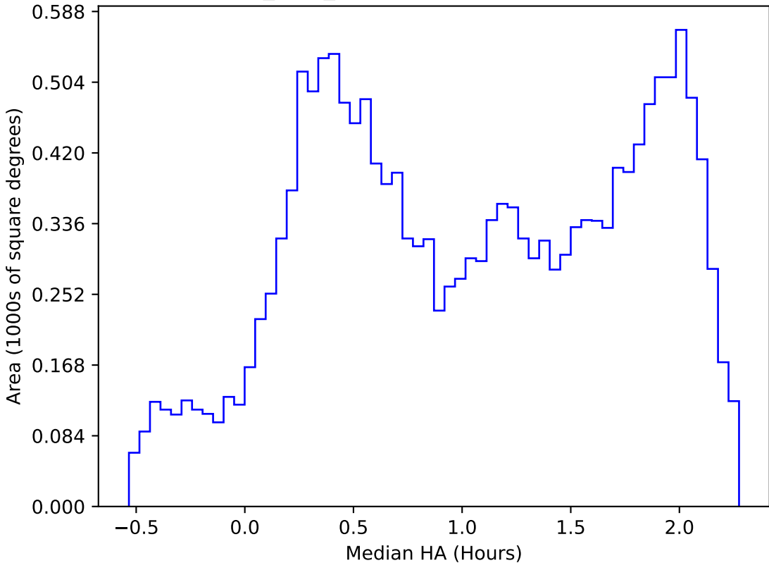
roman_v3.3_10yrs WFD z band: Median HA
