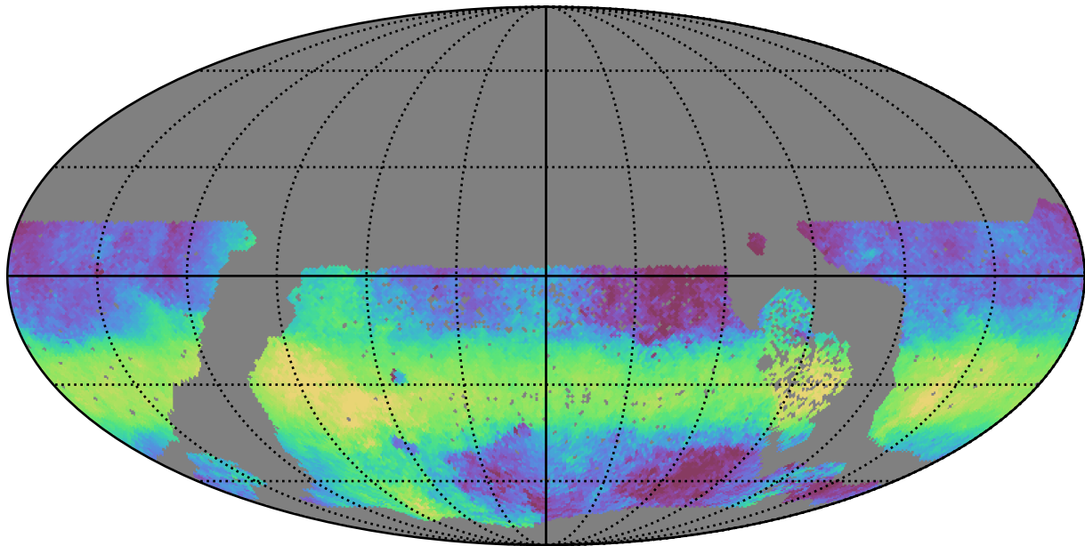
roman_v3.3_10yrs WFD y band: Median HA
