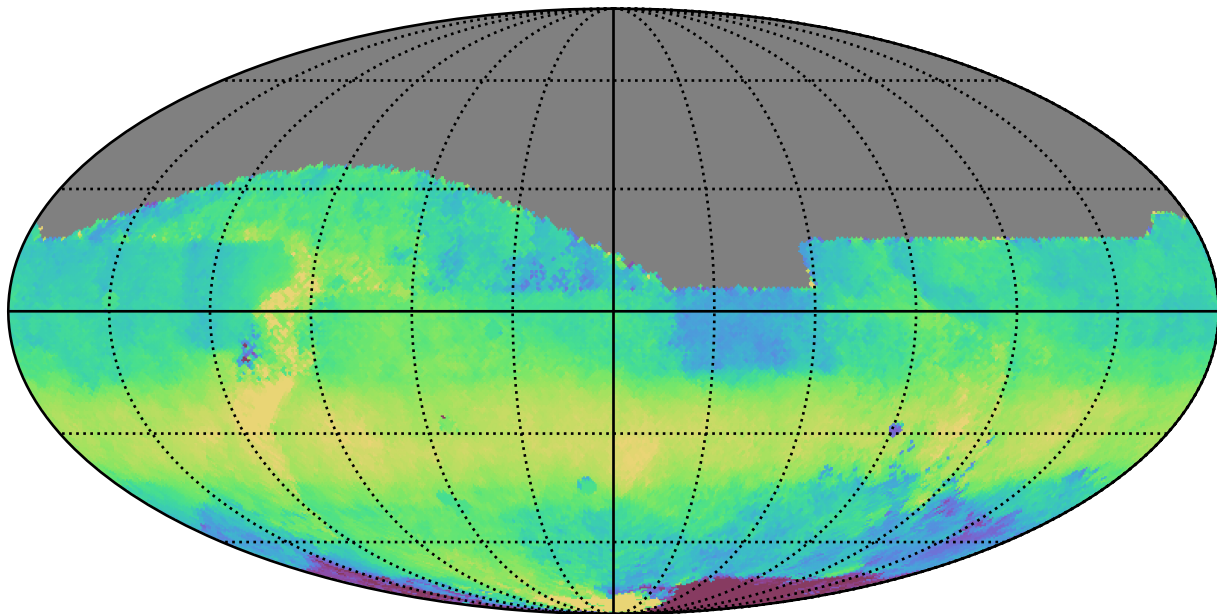
roman_v3.3_10yrs All sky z band: Median HA
