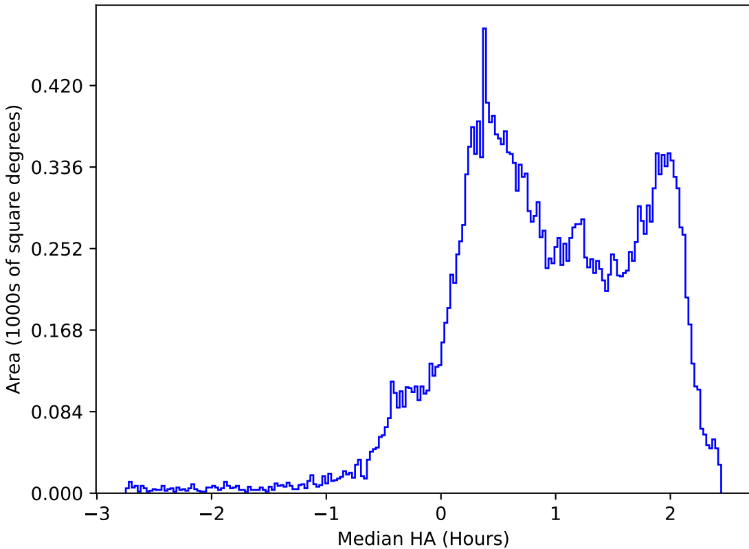
roman_v3.3_10yrs All sky z band: Median HA
