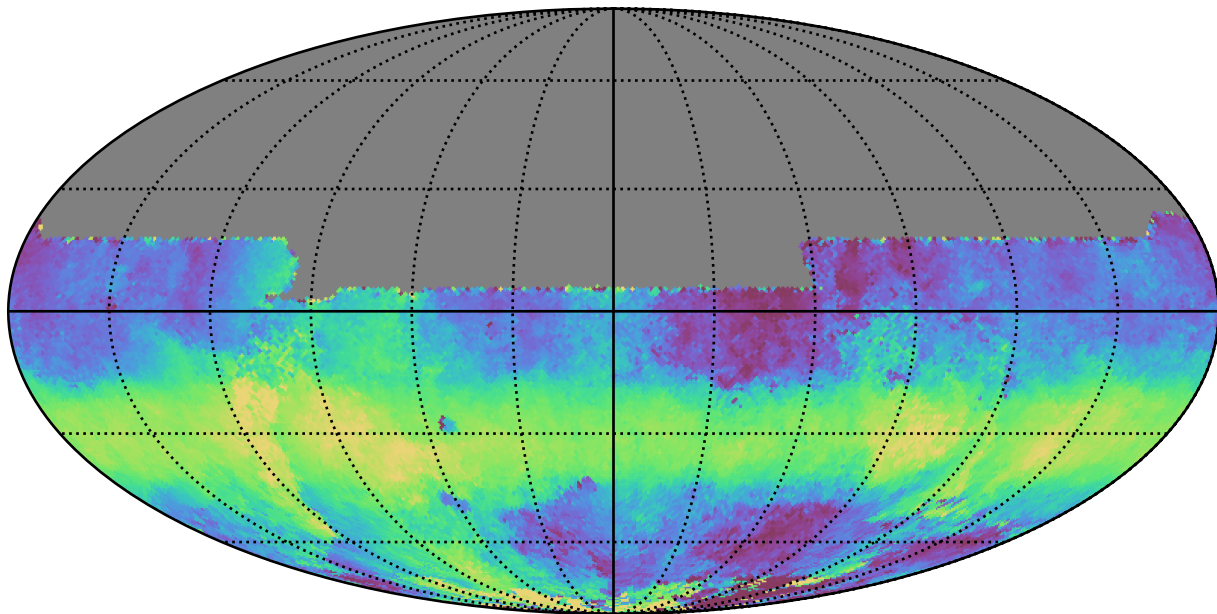
roman_v3.3_10yrs All sky y band: Median HA
