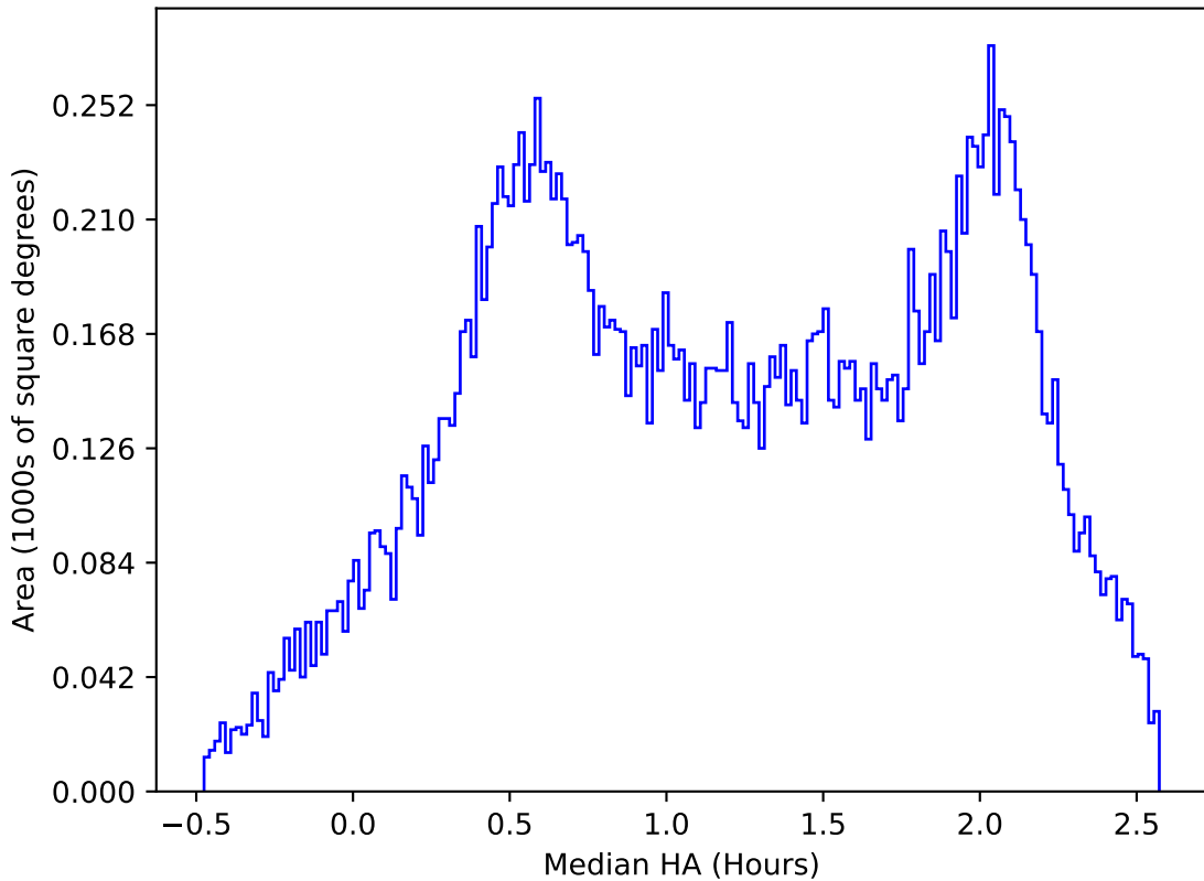
roman_v3.3_10yrs All sky y band: Median HA
