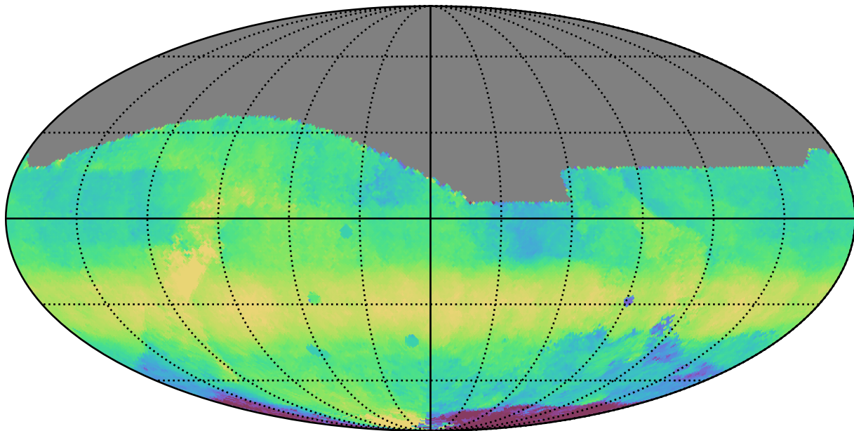
roman_v3.3_10yrs All sky i band: Median HA
