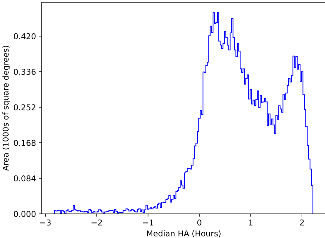
roman_v3.3_10yrs All sky i band: Median HA
