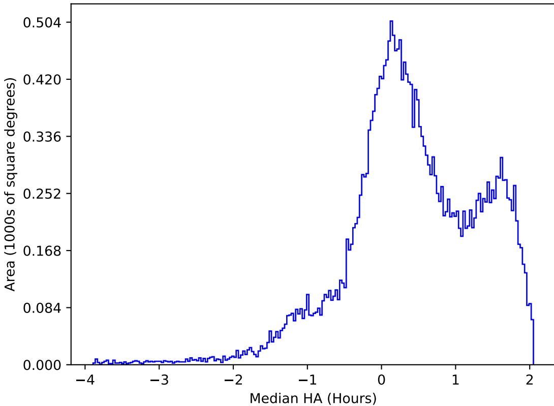
roman_v3.3_10yrs All sky g band: Median HA
