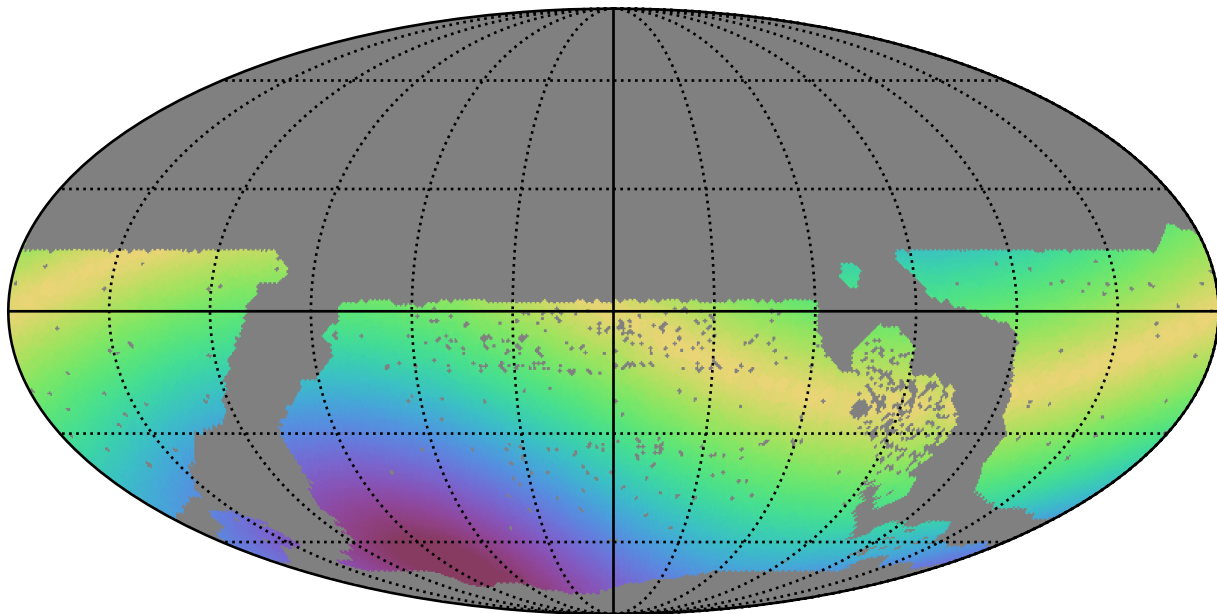
roman_v3.3_10yrs WFD z band: Max solarElong
