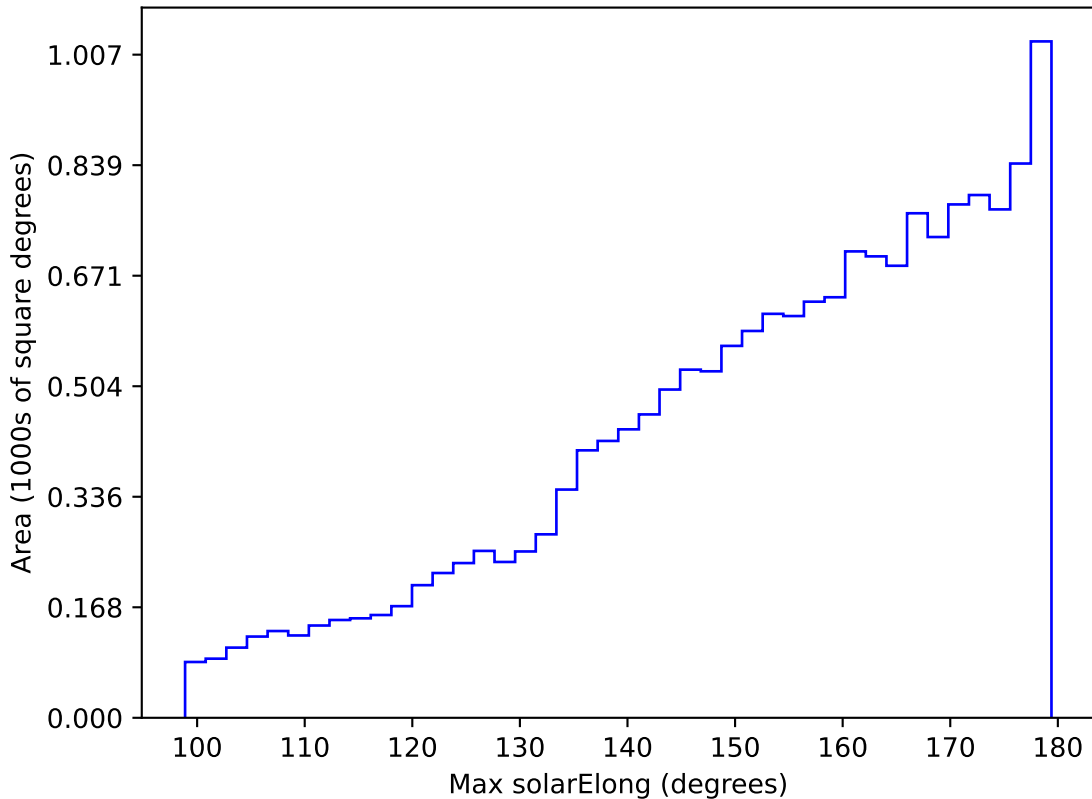
roman_v3.3_10yrs WFD z band: Max solarElong
