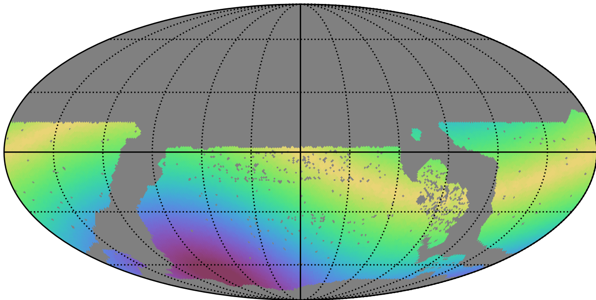
roman_v3.3_10yrs WFD y band: Max solarElong
