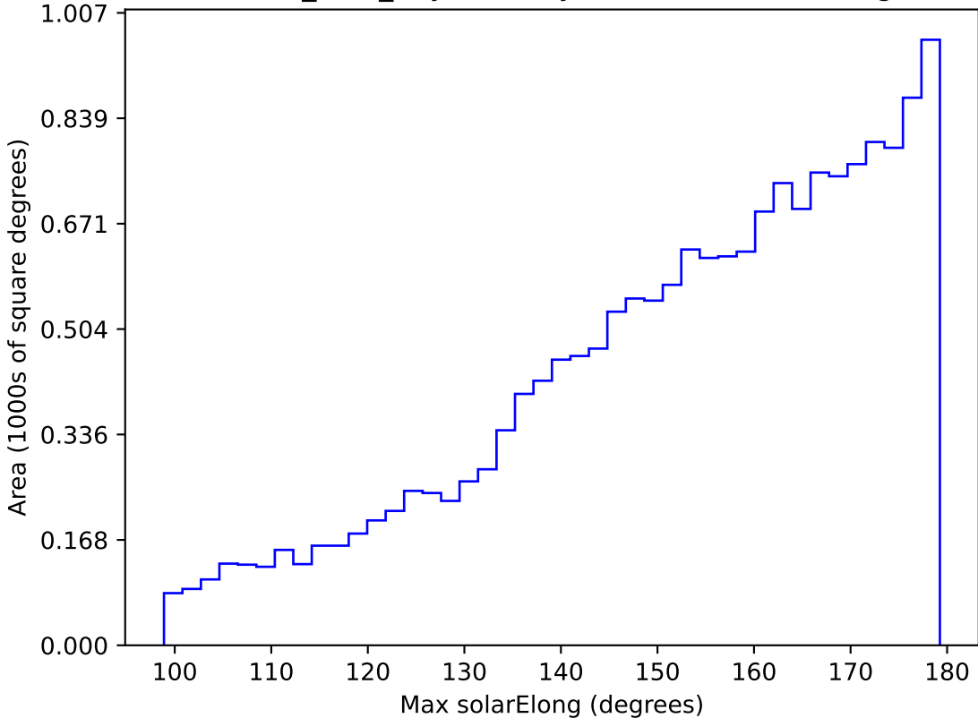
roman_v3.3_10yrs WFD y band: Max solarElong
