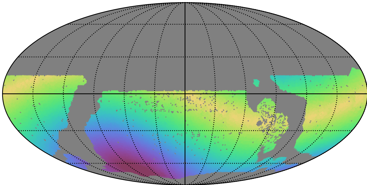
roman_v3.3_10yrs WFD u band: Max solarElong
