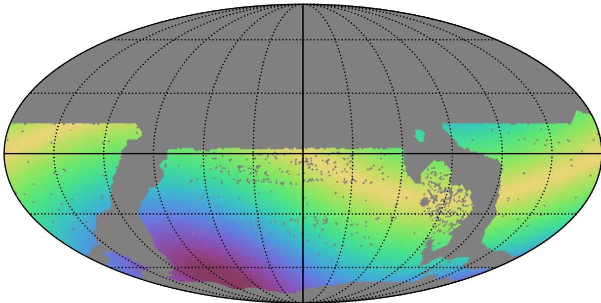
roman_v3.3_10yrs WFD i band: Max solarElong
