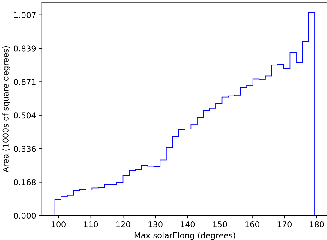
roman_v3.3_10yrs WFD i band: Max solarElong
