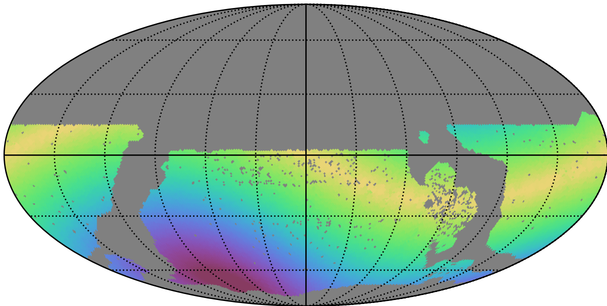
roman_v3.3_10yrs WFD g band: Max solarElong
