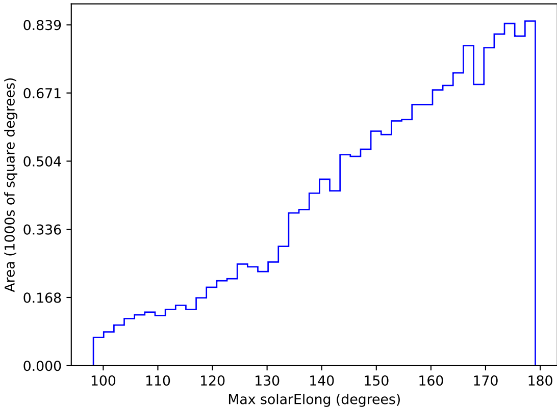
roman_v3.3_10yrs WFD g band: Max solarElong
