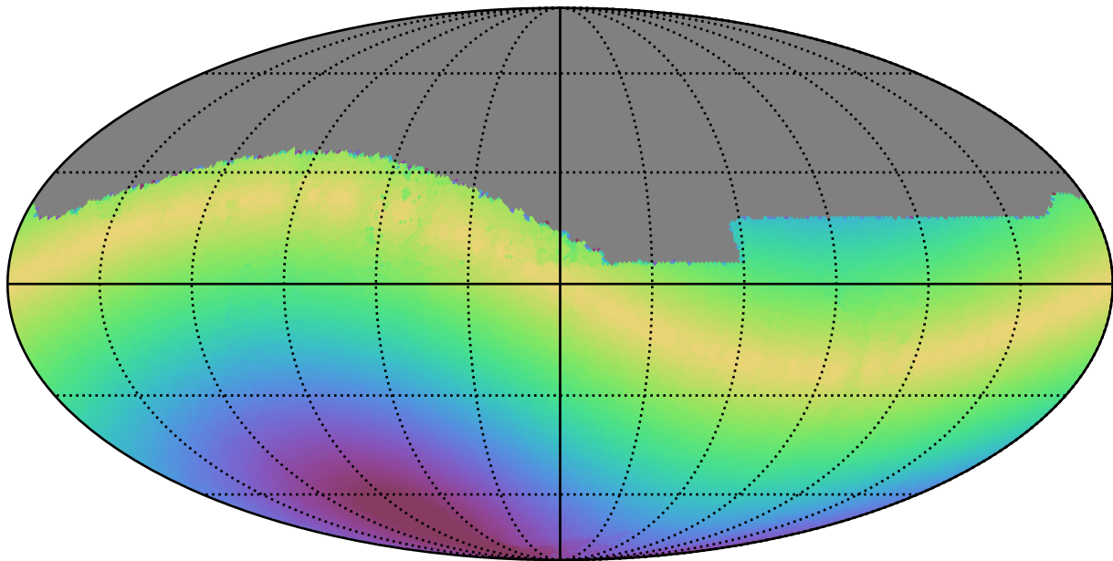
roman_v3.3_10yrs All sky z band: Max solarElong
