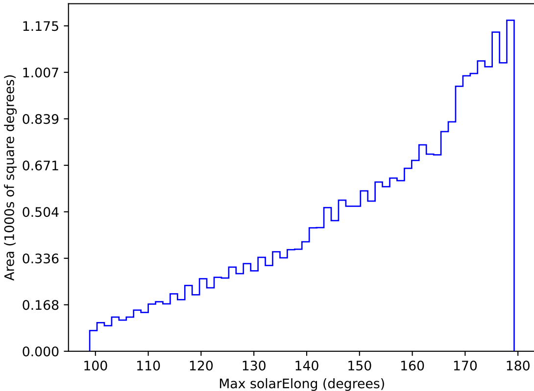
roman_v3.3_10yrs All sky z band: Max solarElong
