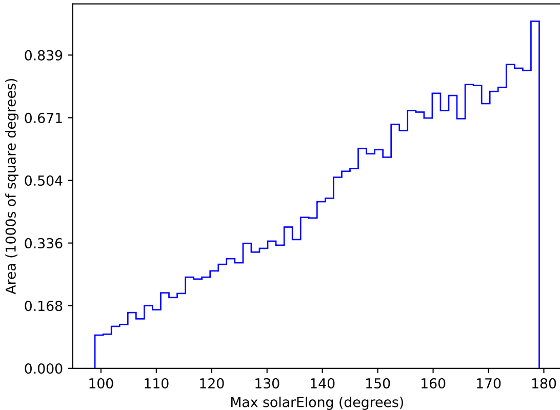
roman_v3.3_10yrs All sky y band: Max solarElong
