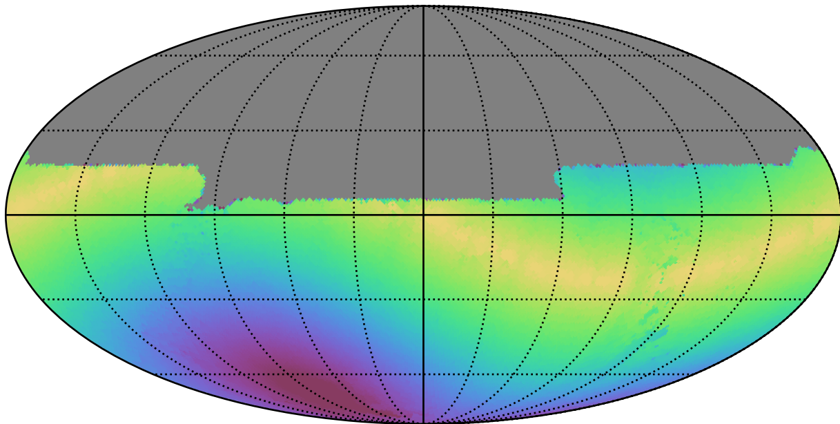
roman_v3.3_10yrs All sky u band: Max solarElong
