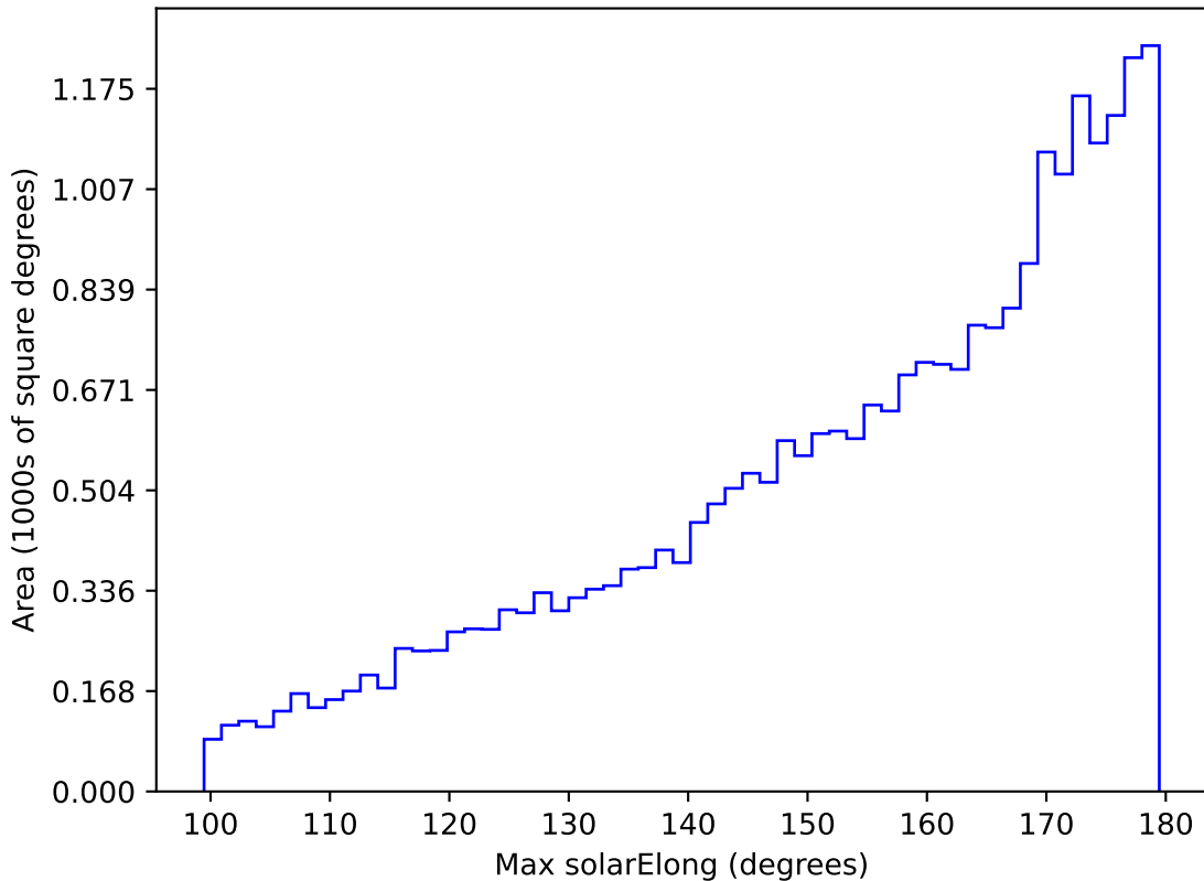
roman_v3.3_10yrs All sky r band: Max solarElong
