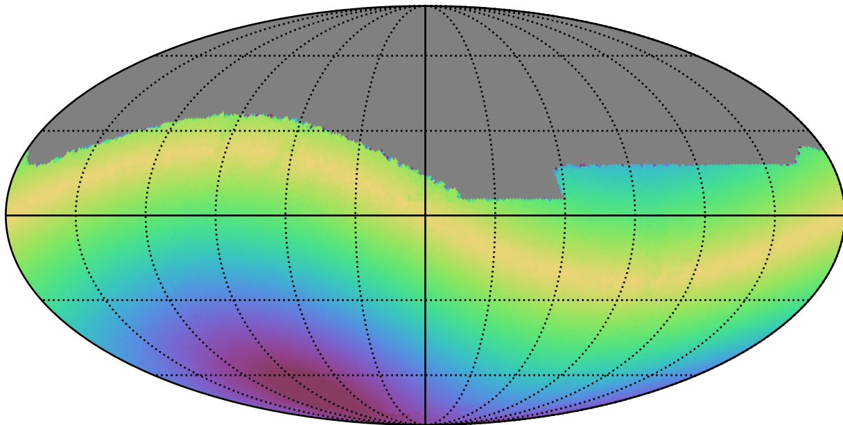
roman_v3.3_10yrs All sky i band: Max solarElong
