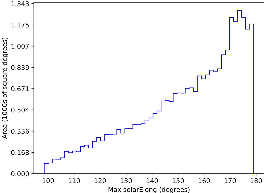
roman_v3.3_10yrs All sky g band: Max solarElong
