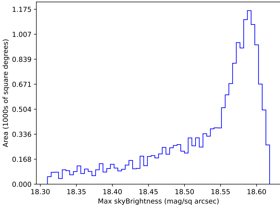
roman_v3.3_10yrs WFD y band: Max skyBrightness
