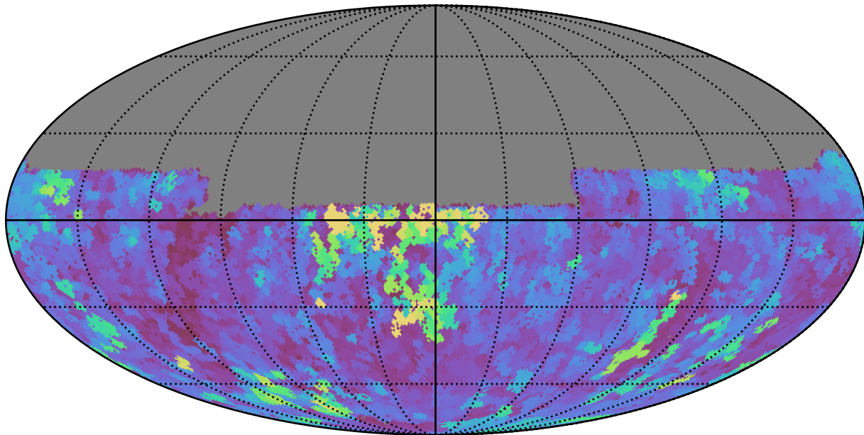
roman_v3.3_10yrs Yr 1 y band: Max seeingGeom
