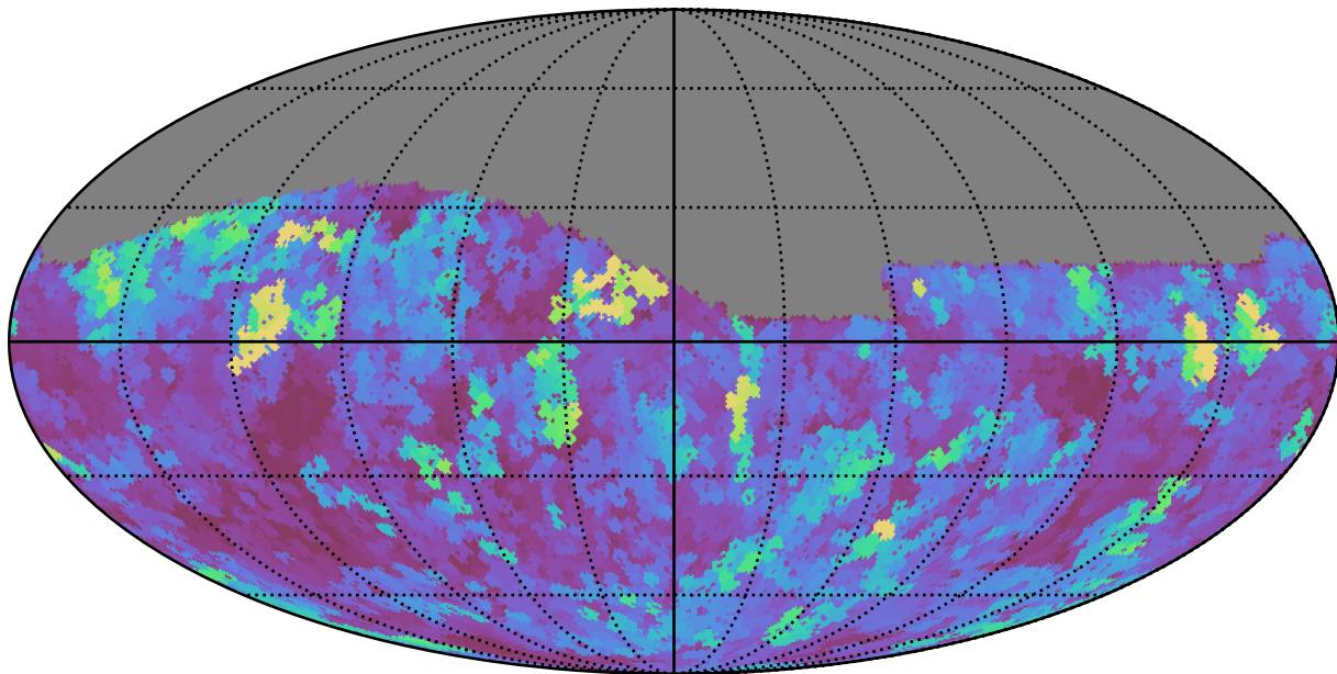
roman_v3.3_10yrs Yr 1 i band: Max seeingGeom
