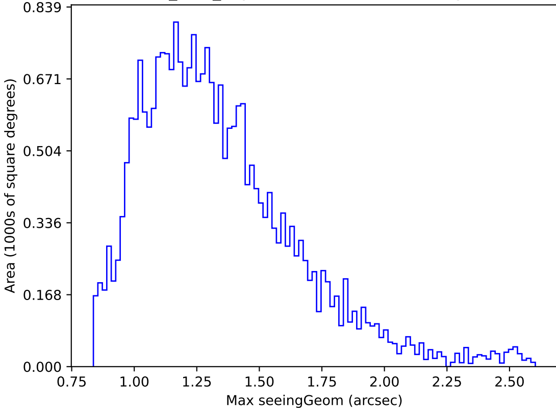
roman_v3.3_10yrs Yr 1 i band: Max seeingGeom
