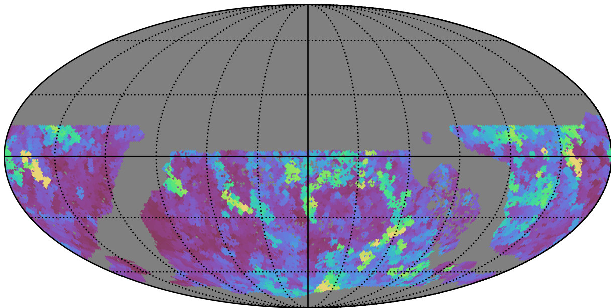
roman_v3.3_10yrs WFD z band: Max seeingEff
