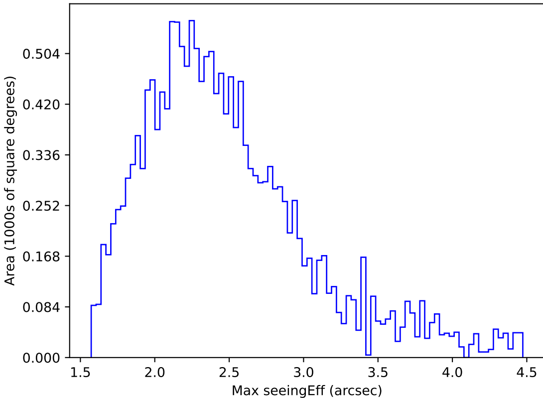
roman_v3.3_10yrs WFD y band: Max seeingEff
