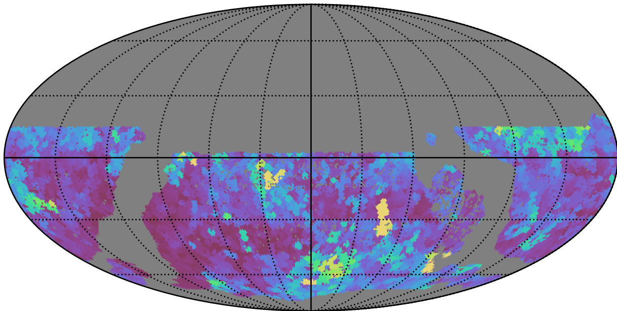
roman_v3.3_10yrs WFD i band: Max seeingEff
