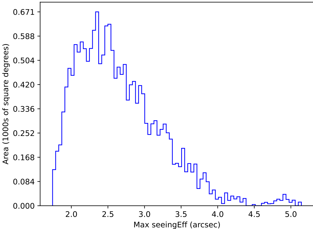
roman_v3.3_10yrs WFD i band: Max seeingEff
