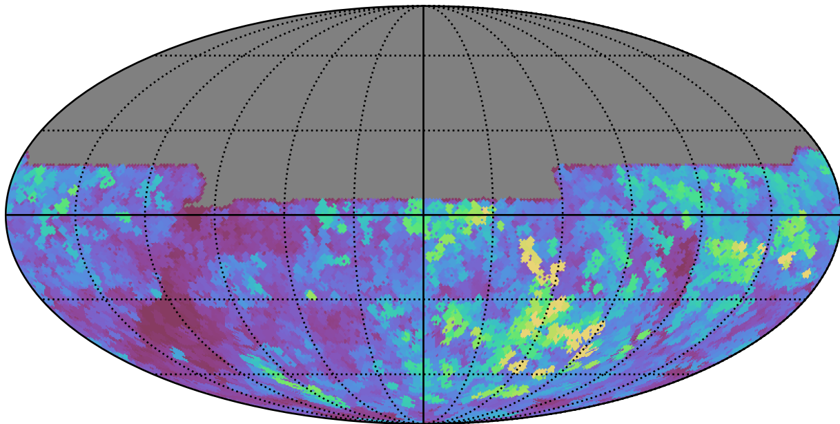
roman_v3.3_10yrs All sky y band: Max seeingEff
