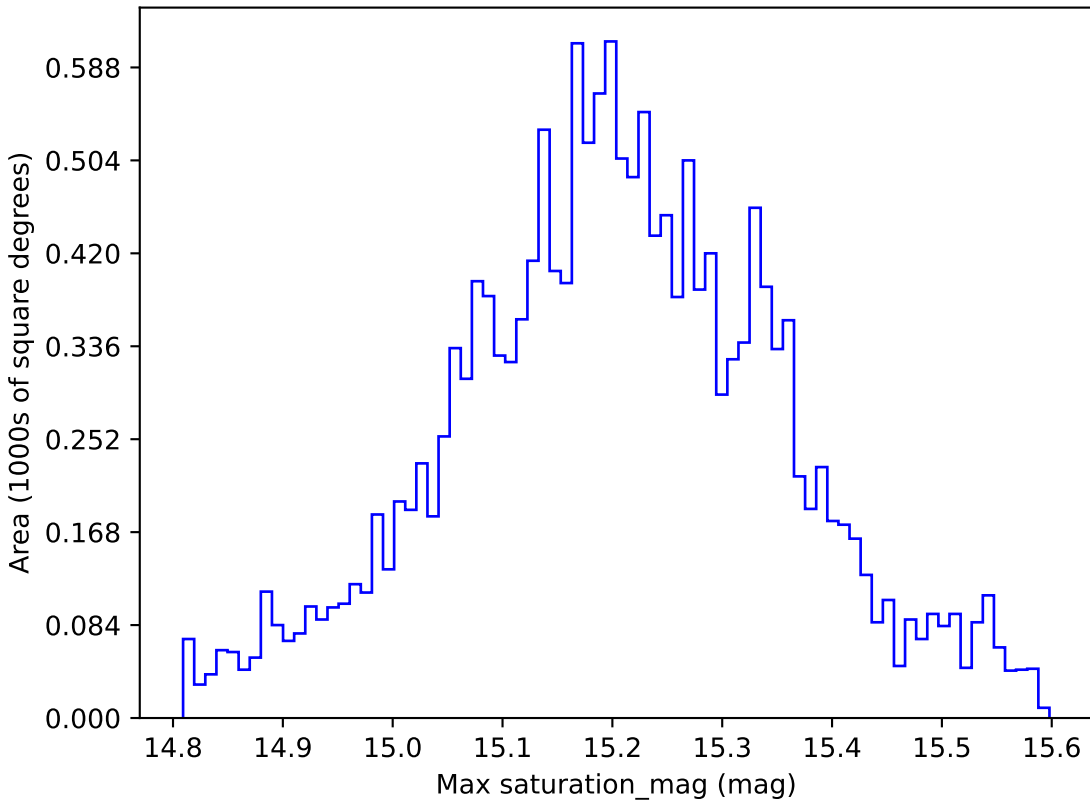
roman_v3.3_10yrs WFD z band: Max saturation_mag
