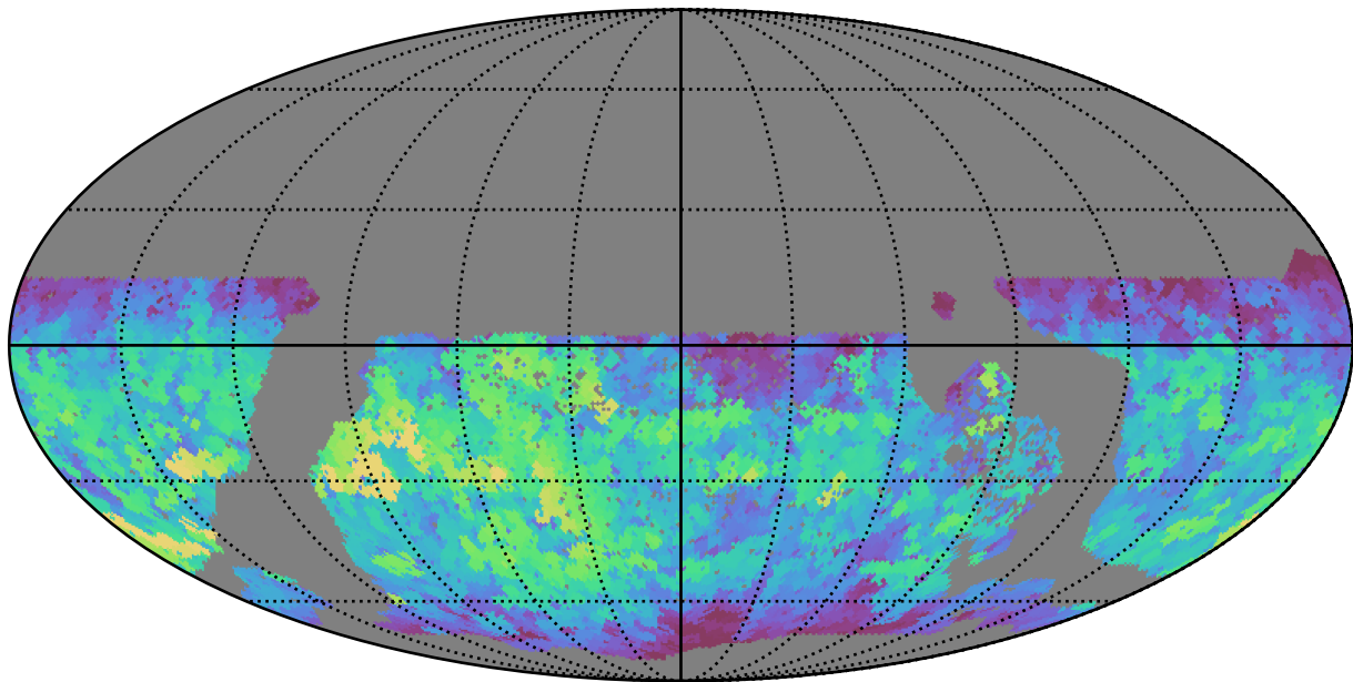
roman_v3.3_10yrs WFD y band: Max saturation_mag
