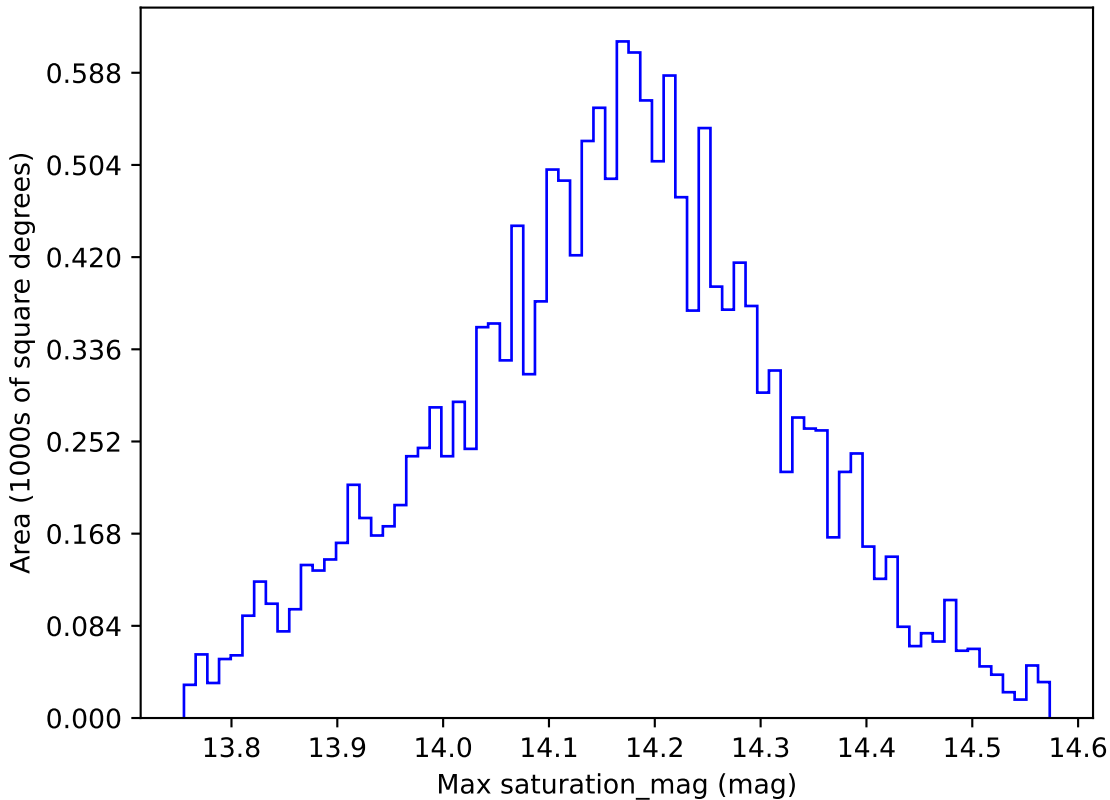
roman_v3.3_10yrs WFD y band: Max saturation_mag
