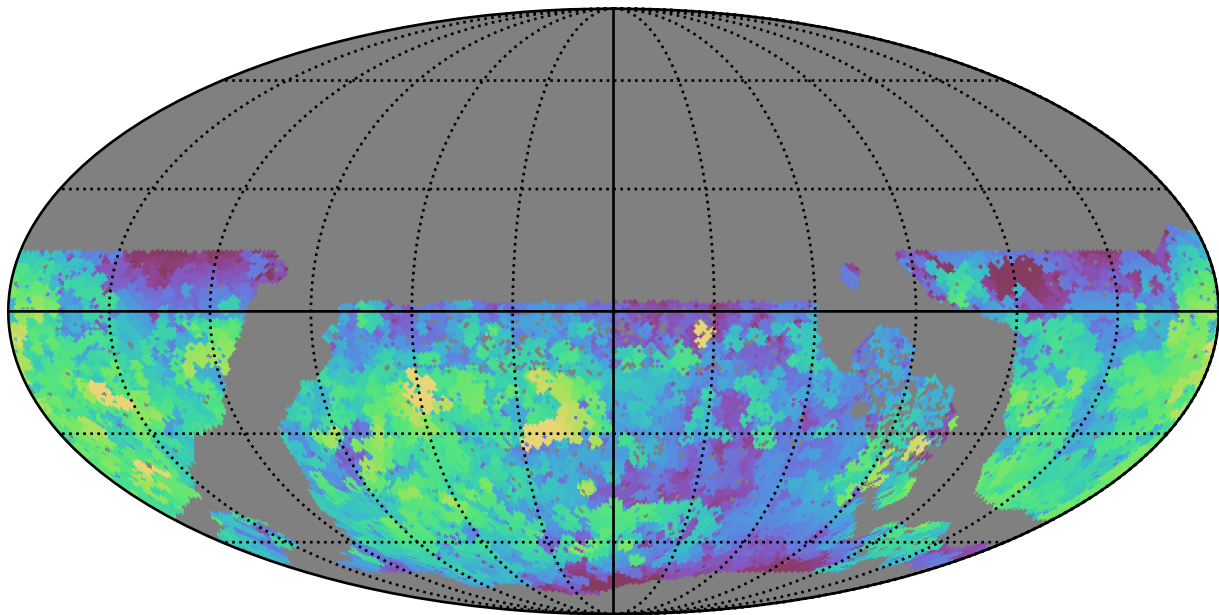
roman_v3.3_10yrs WFD u band: Max saturation_mag
