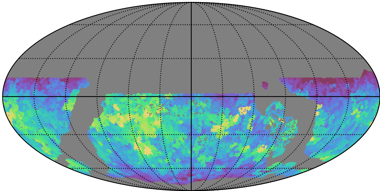
roman_v3.3_10yrs WFD r band: Max saturation_mag
