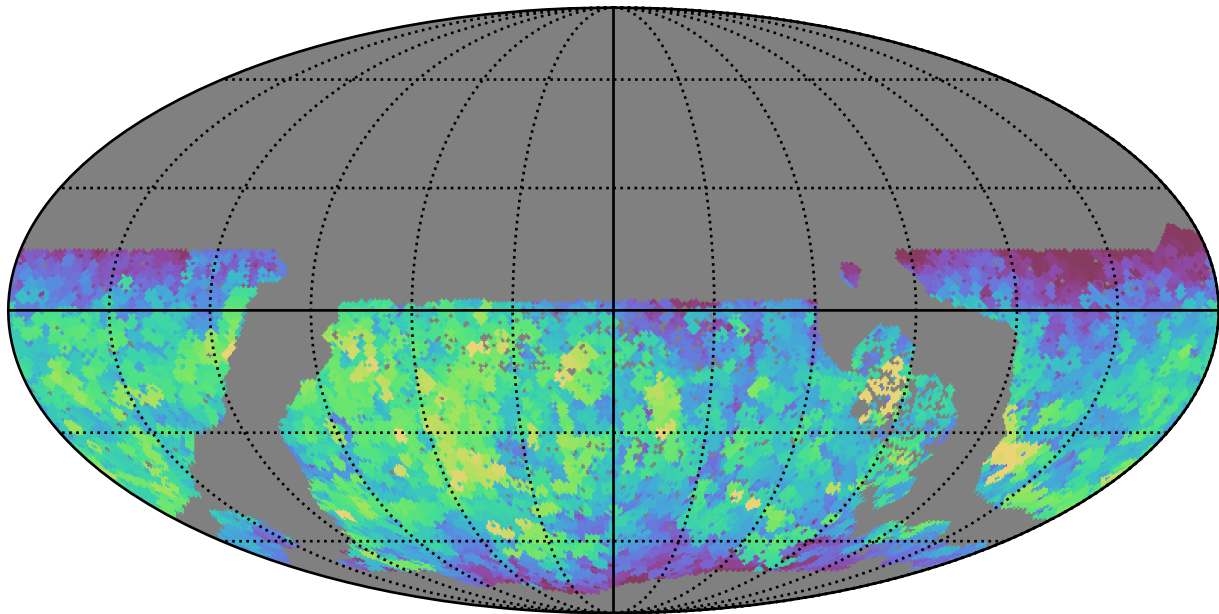
roman_v3.3_10yrs WFD i band: Max saturation_mag
