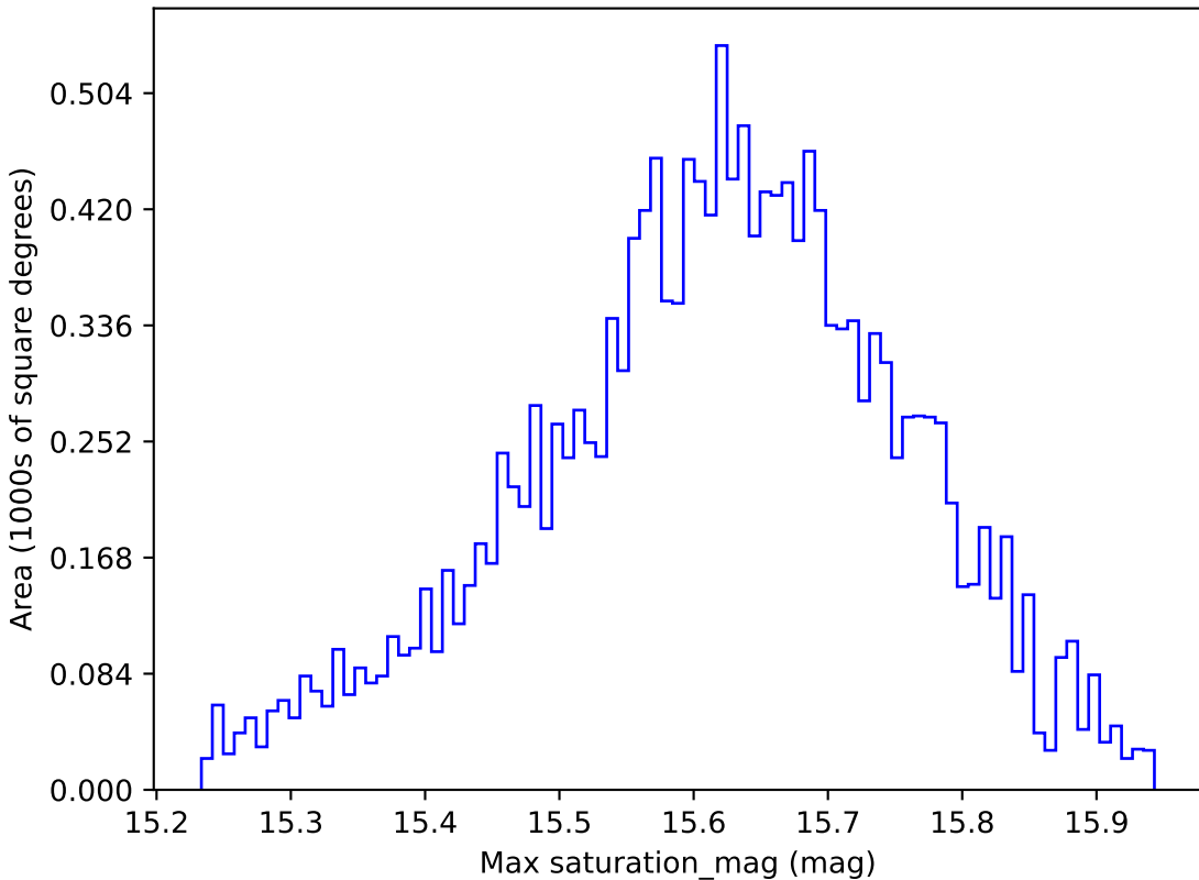
roman_v3.3_10yrs WFD i band: Max saturation_mag
