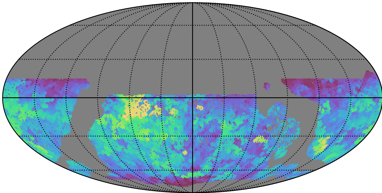
roman_v3.3_10yrs WFD g band: Max saturation_mag
