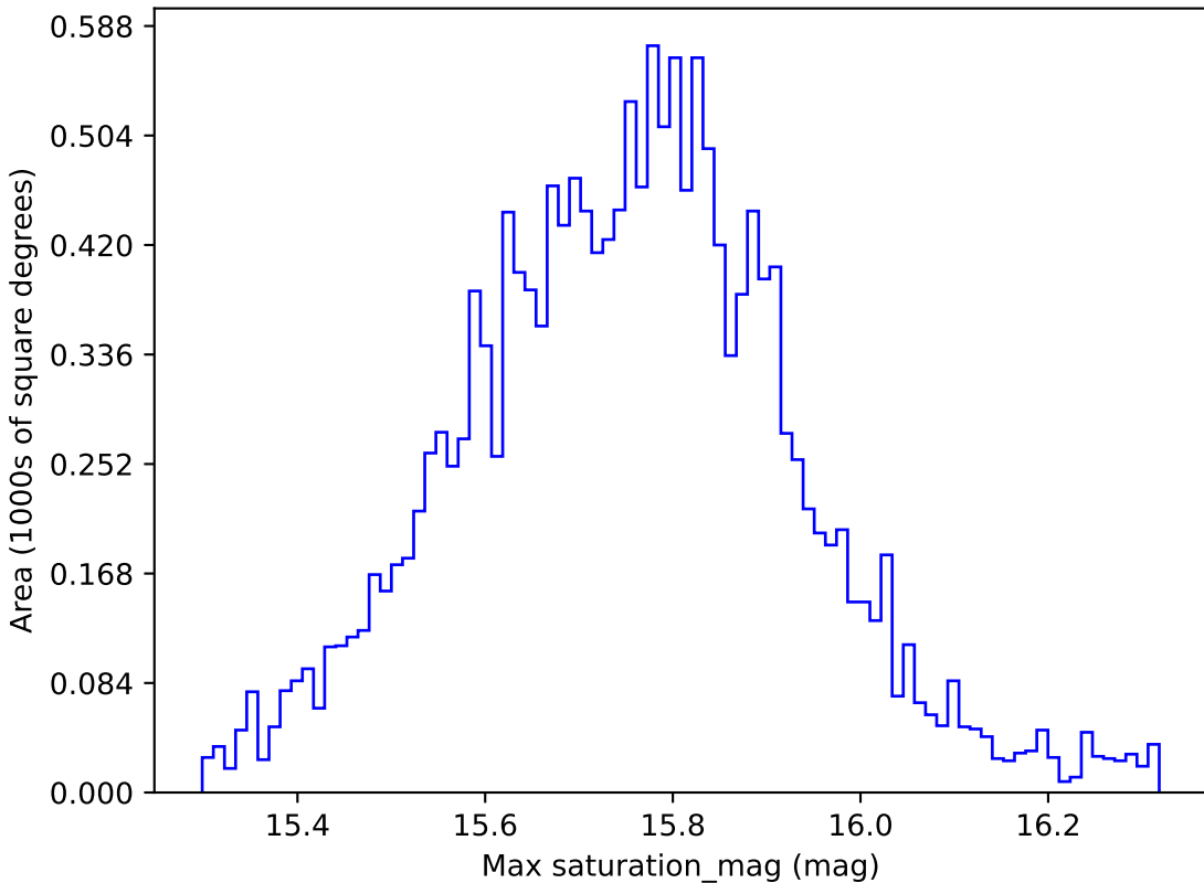
roman_v3.3_10yrs WFD g band: Max saturation_mag
