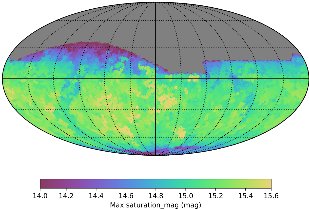
roman_v3.3_10yrs All sky z band: Max saturation_mag
