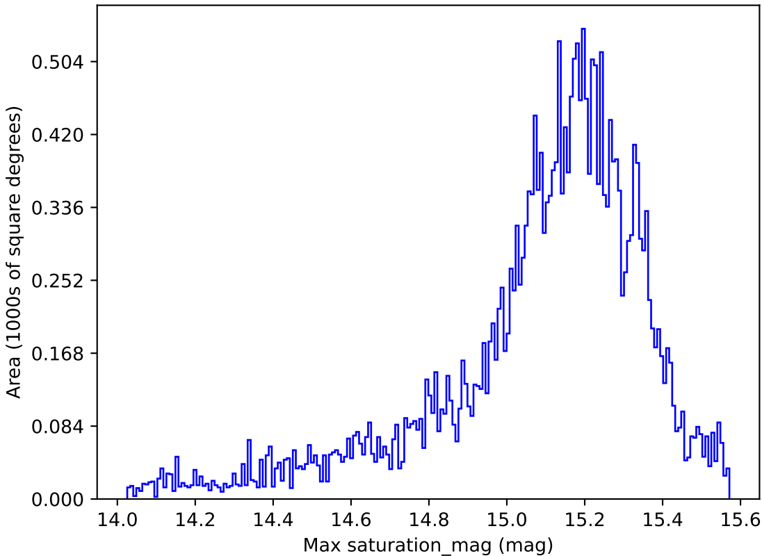
roman_v3.3_10yrs All sky z band: Max saturation_mag
