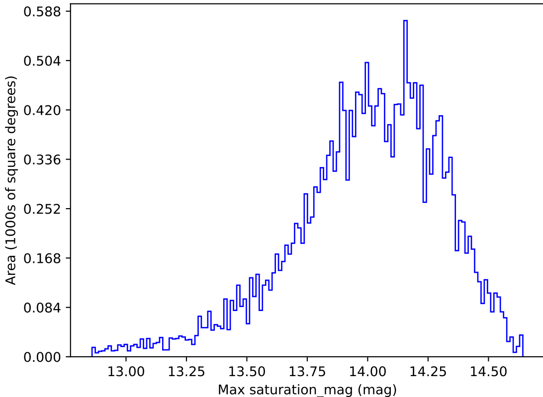
roman_v3.3_10yrs All sky u band: Max saturation_mag
