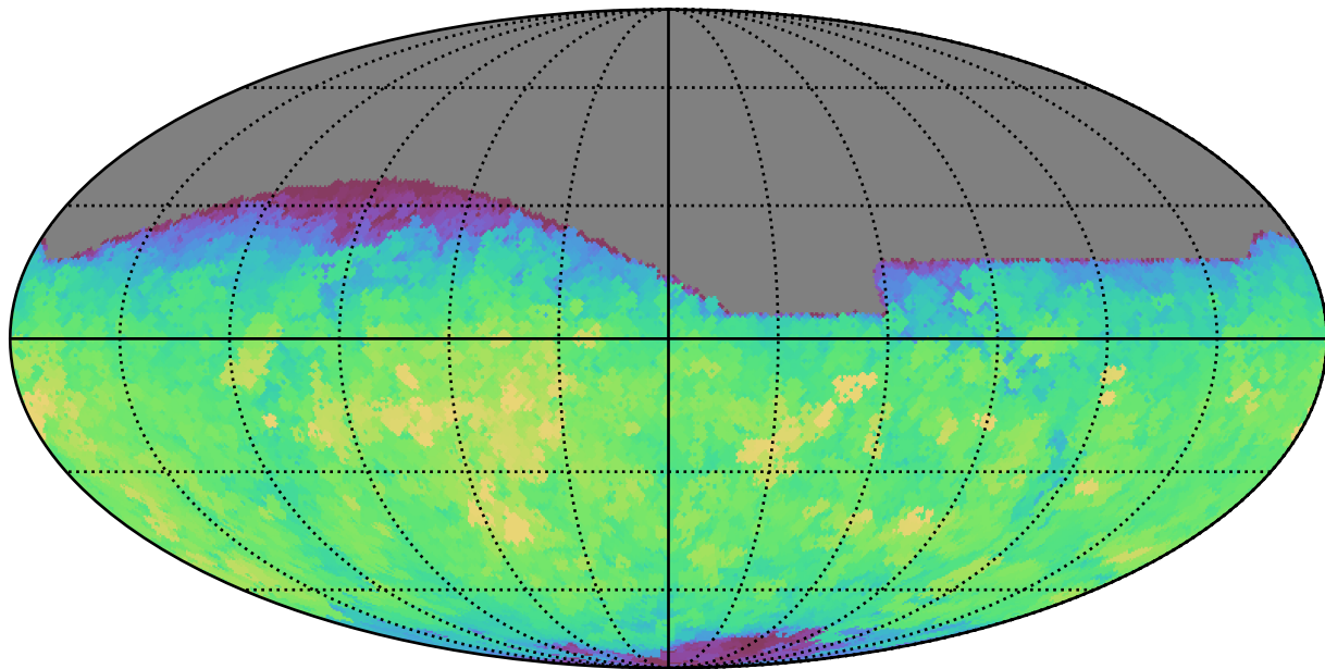
roman_v3.3_10yrs All sky r band: Max saturation_mag
