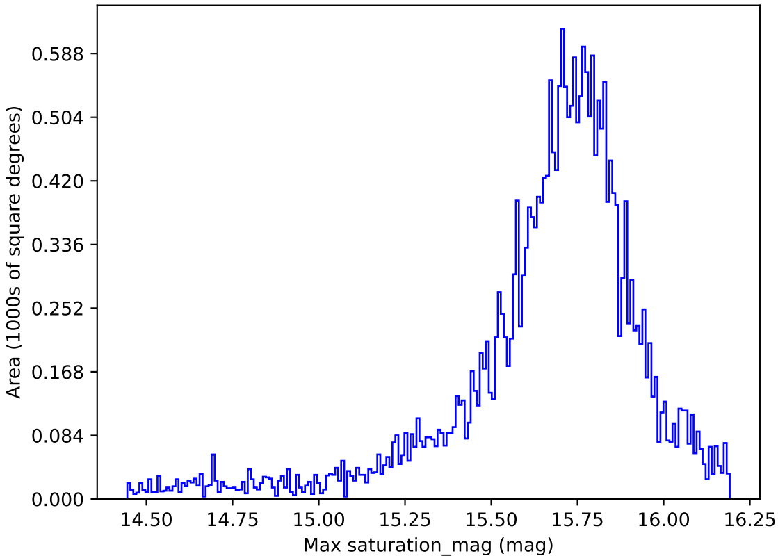
roman_v3.3_10yrs All sky r band: Max saturation_mag
